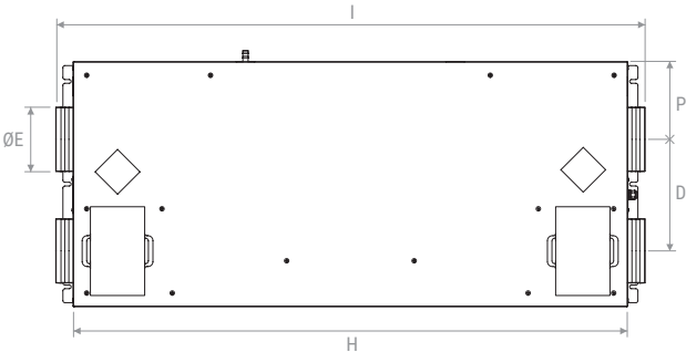
Vista dal basso | Bottom View
