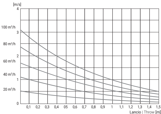
100 / 125 VELOCITÀ | VELOCITY m/s
