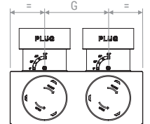
Vista superiore | Top view
