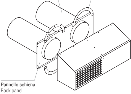
Canali di uscita del muro Ducts coming out of the wall Ghigliottine per adattamento circonferenza dei canali Ghillottines for circumference adaption of the ducts
